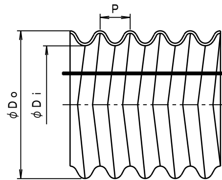
φ30、φ40、φ50形状図
