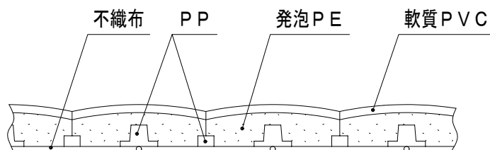
断面図
